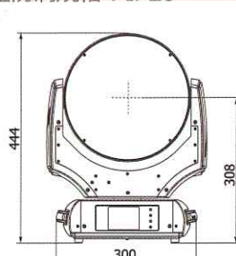
LEDWash600X 外観図
