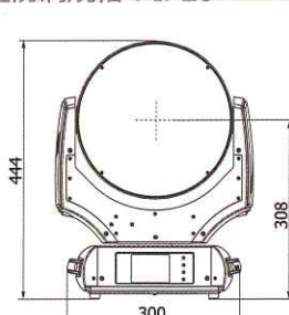
LEDWash600X 外観図
